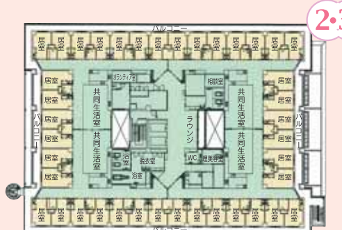
【特別養護老人ホーム・老人短期入所施設平面図】
